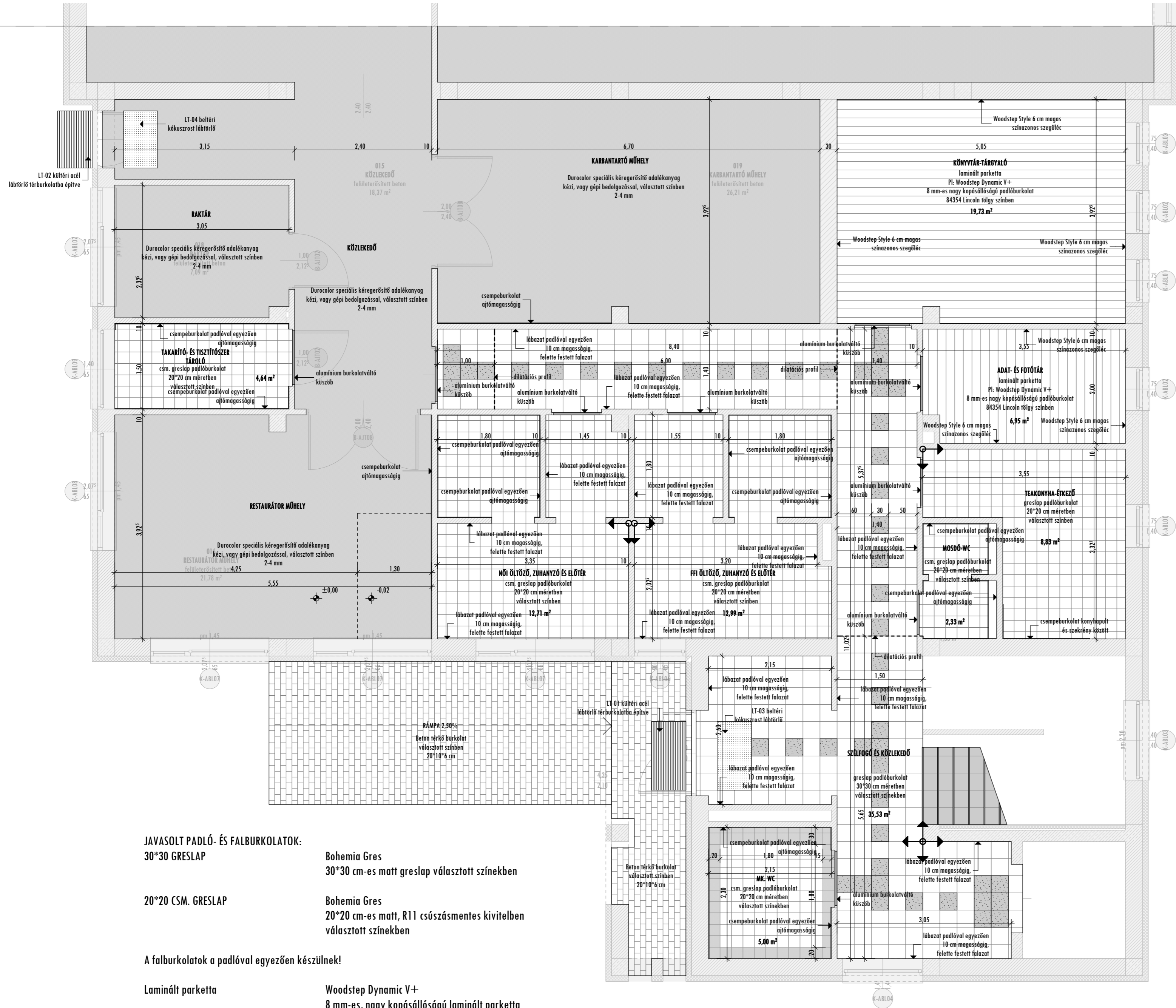
FÖLDSZINTI BURKOLÁSI TERV
